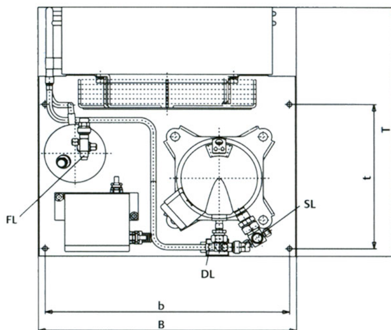
с компрессором ZF
