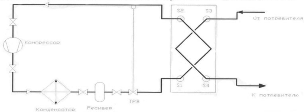
Гидравлическая схема холодильной установки типа ХМП-ОЖ-*-С
