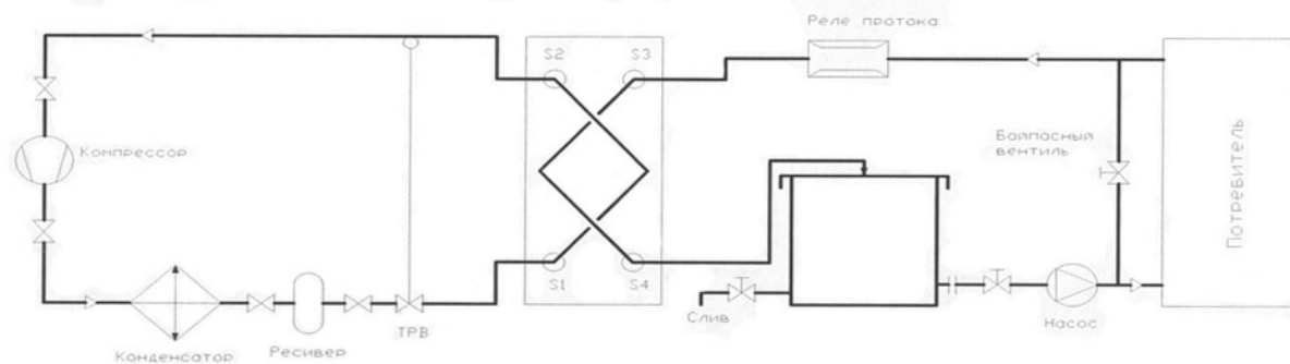
Гидравлическая схема холодильной установки типа ХМП-ОЖ-*-А
