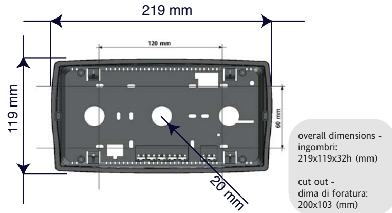
FIG. 9 Dimensions-Dimensioni
