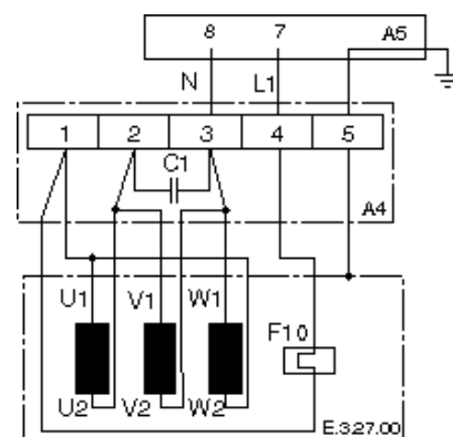
Рис.19 Однофазное соединение
