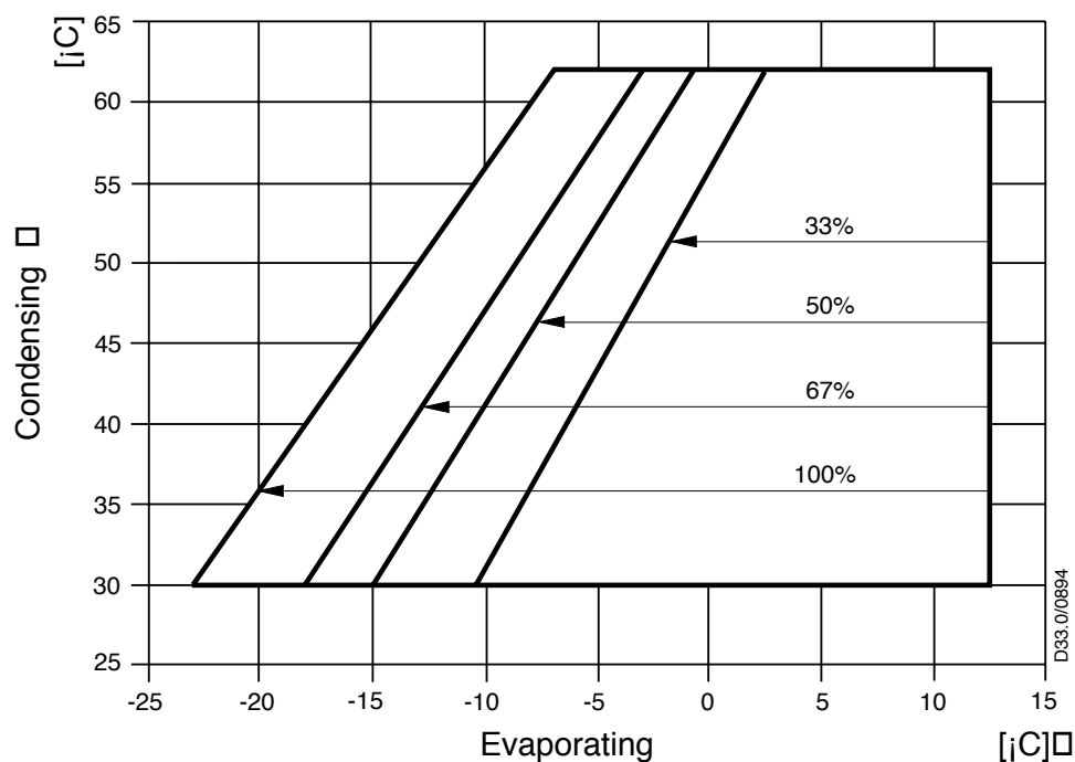
Диаграмма 1 Температура всасываемого газа 25°C
