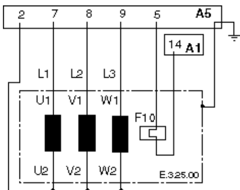
Рис.17 Соединение «звезда»
